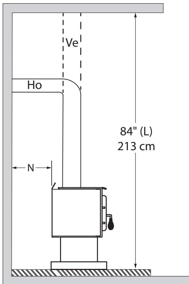
Figure 10: Dégagements - Plafond
